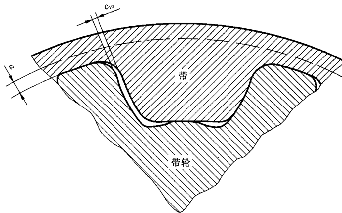
图 11 ZS 和 YS 型带与带轮的间隙(见表 11)
