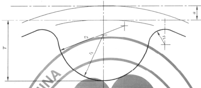
图 7 ZH 和 YH 型轮槽尺寸(见表 9)
