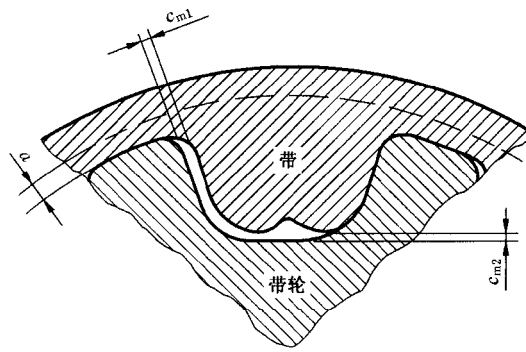
图 9 ZR 和 YR 型带与带轮的间隙(见表 10)
