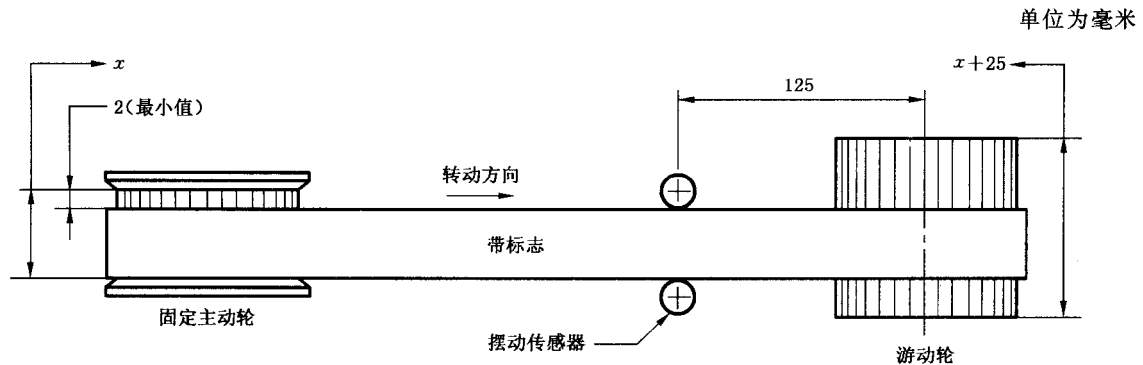
图 12 横向摆动测量装置(俯视图)
