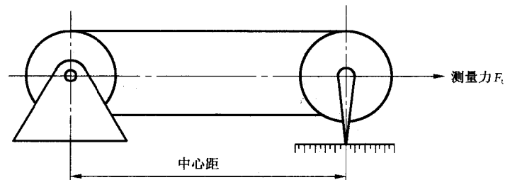
图 5 节线长测量装置
