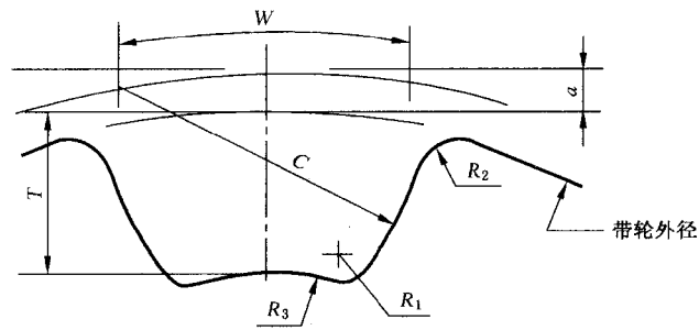
图 10 ZS 和 YS 型轮槽尺寸(见表 11)
