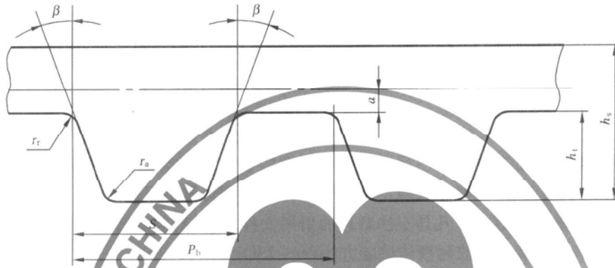
图1 ZA型和ZB型梯形齿带齿公称尺寸(侧视图)
