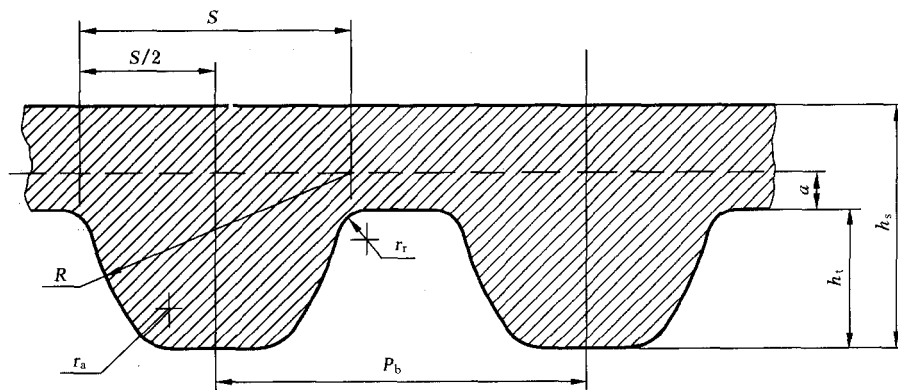
图 4 ZS型和 YS型带齿公称尺寸(侧视图)
